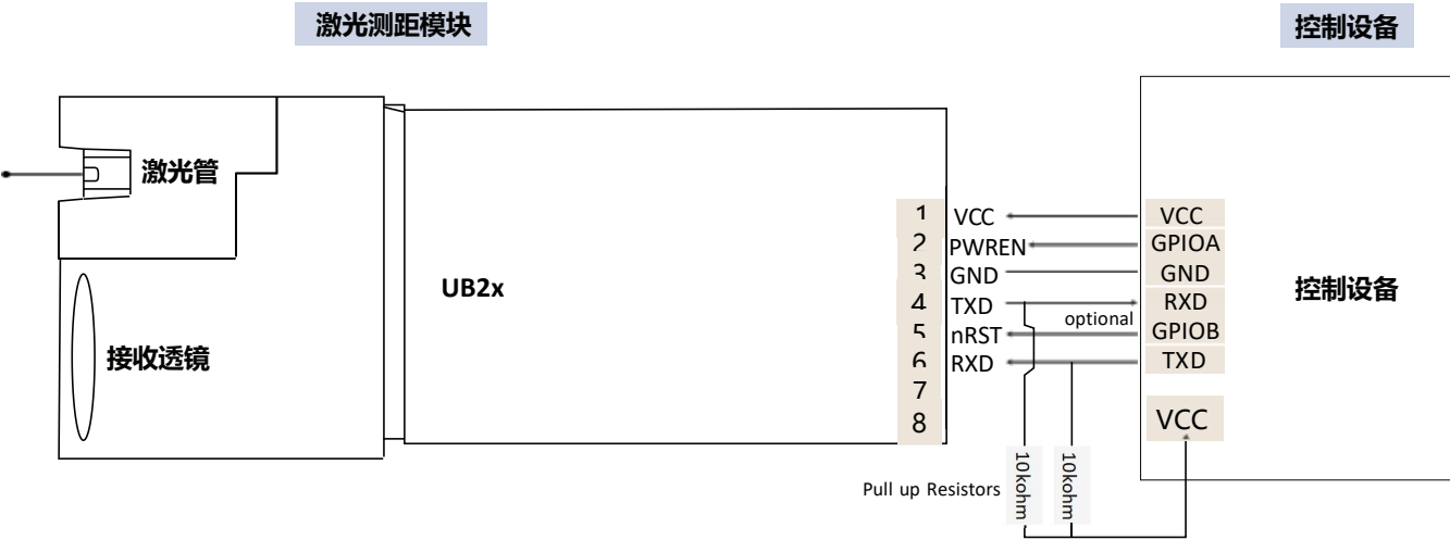
图4-1 模块引脚布局及推荐连线
