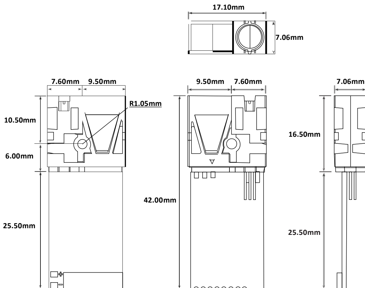
图2-2 模块结构尺寸图
