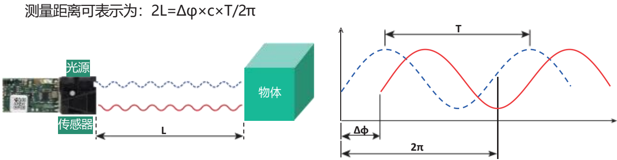
图1-1 激光模块基本原理图
