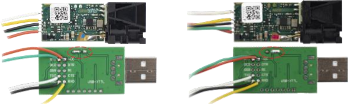
图5-2 半孔焊接
